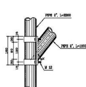
DET. 7 SC 1:5
