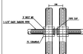
DET. 6 SC 1:5
